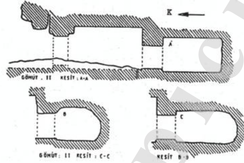
2. Mezar Kesiti (Çizim: Nevzat Çevik)
