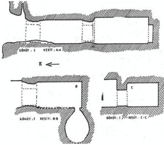
1. Mezar Kesiti (Çizim: Nevzat Çevik)
